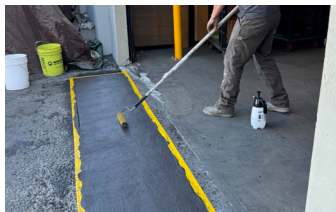
Utilización del rodillo de textura GST para la colocación final.
