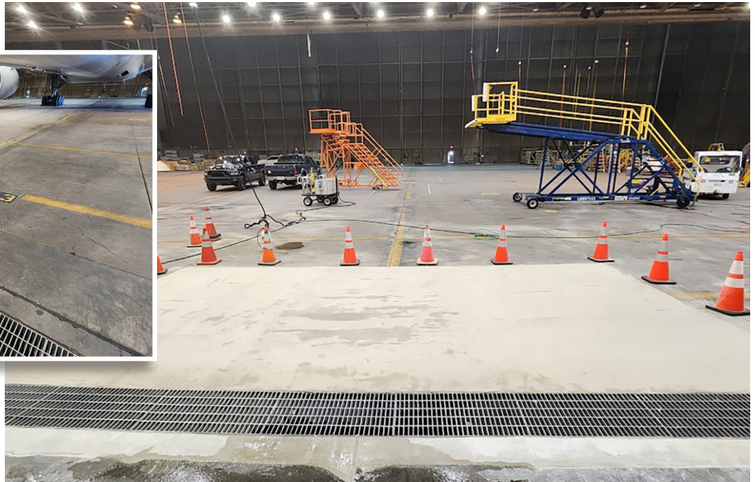
Foto que muestra daños extensos en el concreto alrededor de los desagües, incluida una depresión de 'carga puntual' de 3" en el área de estacionamiento en el tren de morro del avión.
