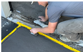
Acabado de bordes con una llana.
